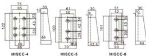
電纜夾
